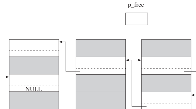
图 6-4 多块中的自由节点链表
