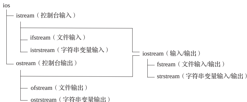
图 8-1 I/O 类库中主要的类以及它们之间的关系
