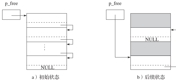
图 6-3 单块中的自由节点链表
