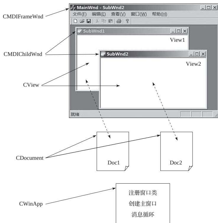
图 11-2 一个多文档应用程序中包含的对象以及它们所属的 MFC 基类
