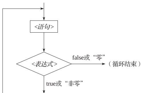
图 3-5 do-while 语句的含义
