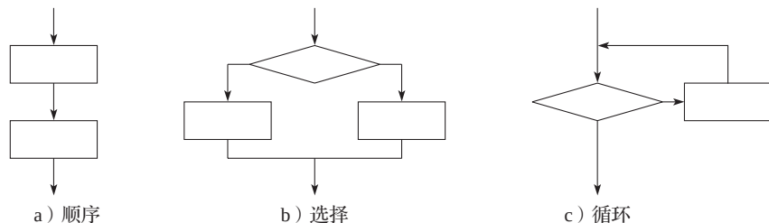
图 3-7 结构化程序的三种基本结构
