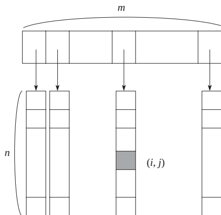
图 5-3 m 行 n 列的动态二维数组
