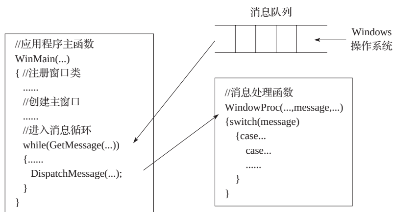
图 11-1 Windows 应用程序的基本框架
