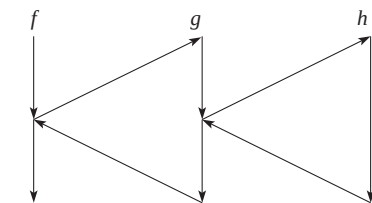
图 4-3 函数的嵌套调用及逐层返回
