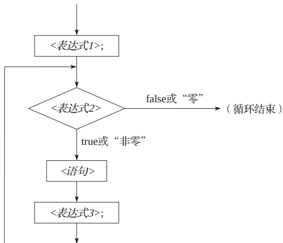
图 3-6 for 语句的含义
