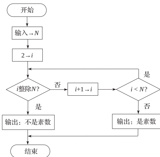
图 3-1 程序流程图示例
